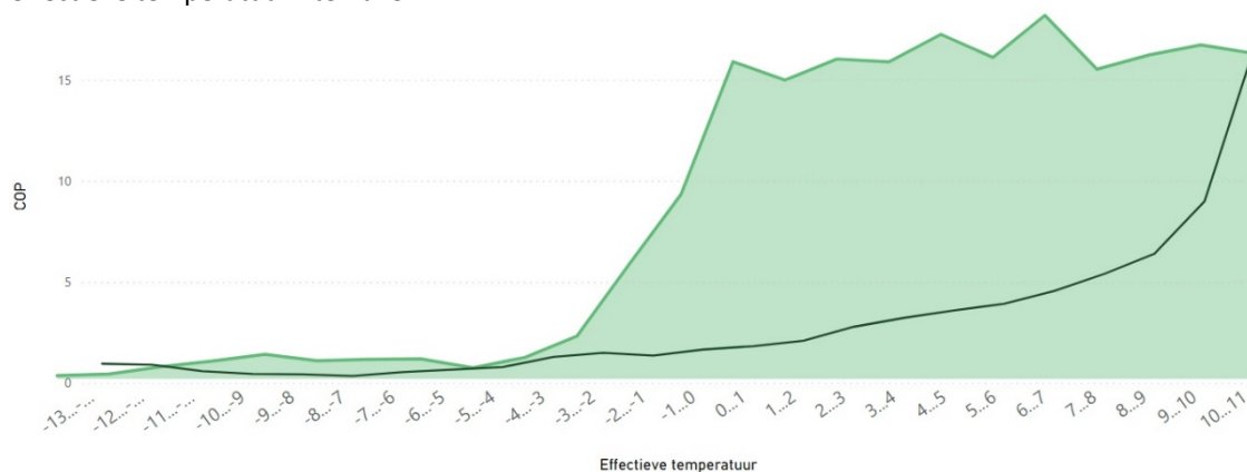
Figuur 19 - COP als functie van de effectieve buitentemperatuur. Op de achtergrond de frequentie waarmee de betreffende effectieve buitentemperatuur is voorgekomen in 2020-2021.
