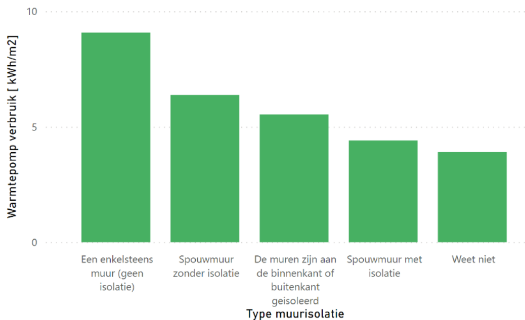
Figuur 3 - Gemiddeld warmtepompverbruik [kWh/m2] per type muurisolatie.
