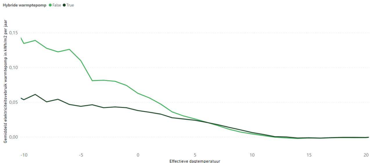
Figuur 21 - Gemiddeld elektriciteitsverbruik van de warmtepomp in kWh/m 2 per jaar uitgezet tegen de effectieve dagtemperatuur.
